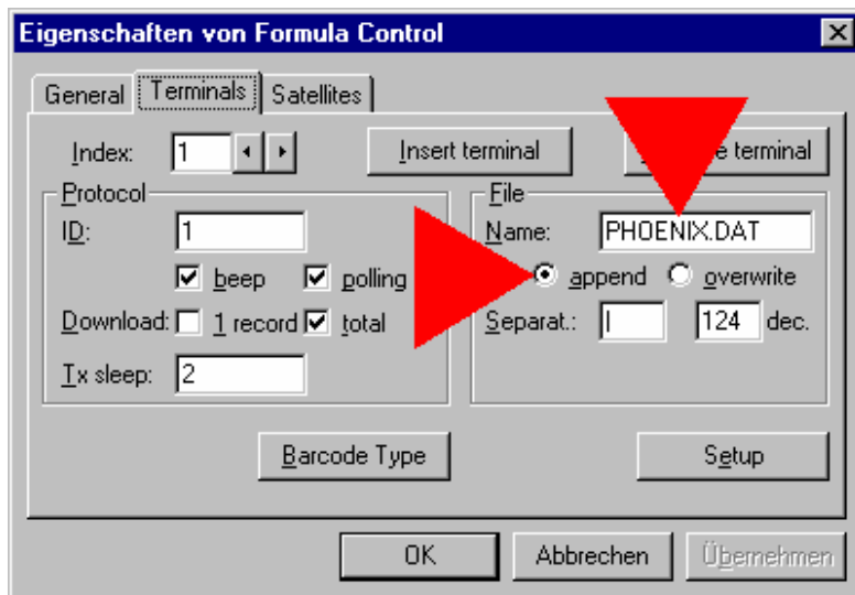
Abb. 45 Konfigurationsdaten
