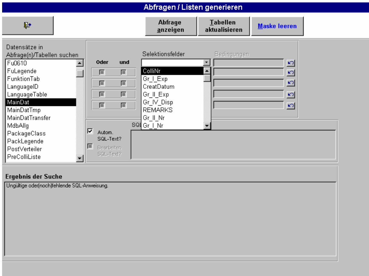
Abb. 40 Datenselektion
