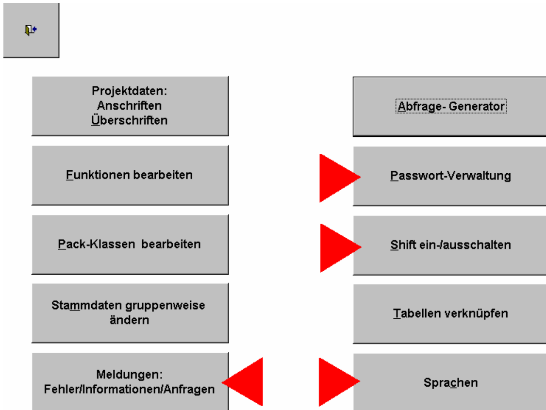
Abb. 9 Systemdaten
