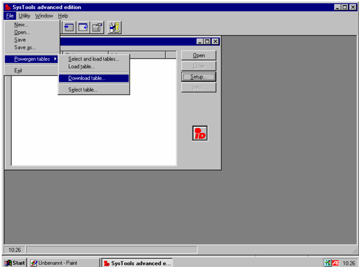
Abb. 46 Datenübernahme
