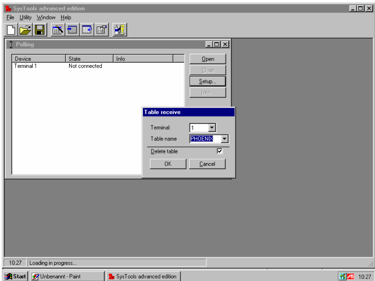
Abb. 47 Tabellenübernahme
