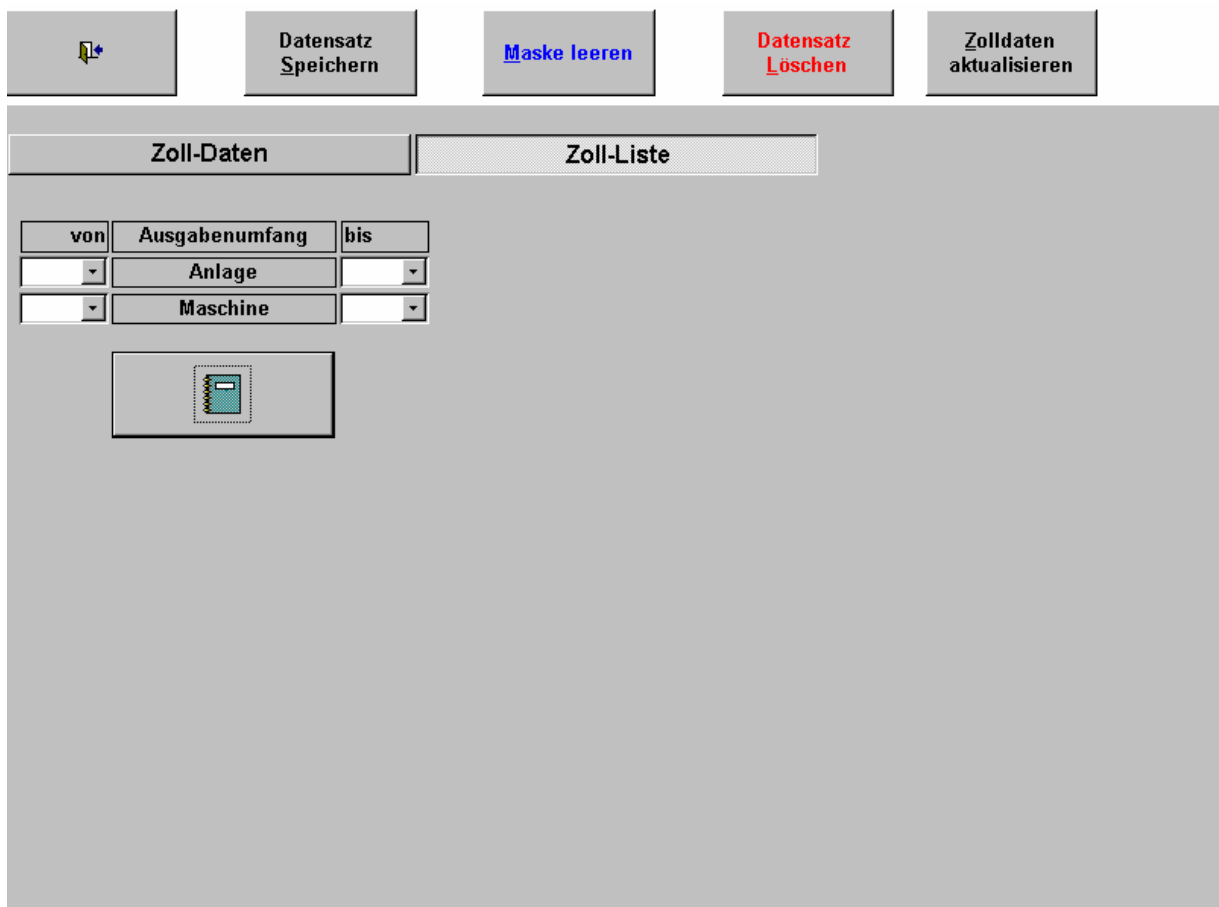
Abb. 38 Zolllistenausgabe
