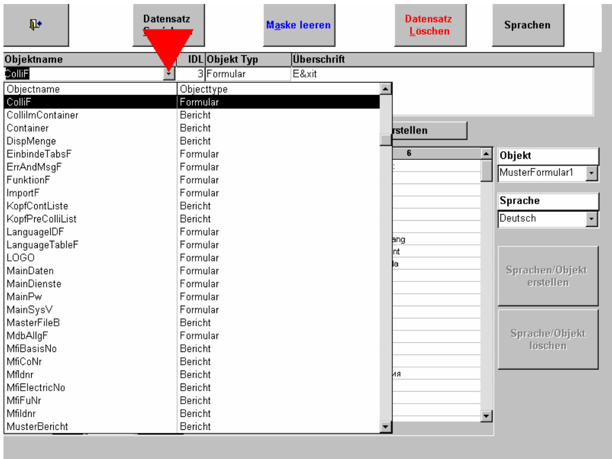
Abb. 13 Sprachverwaltung / Objektauswahl
