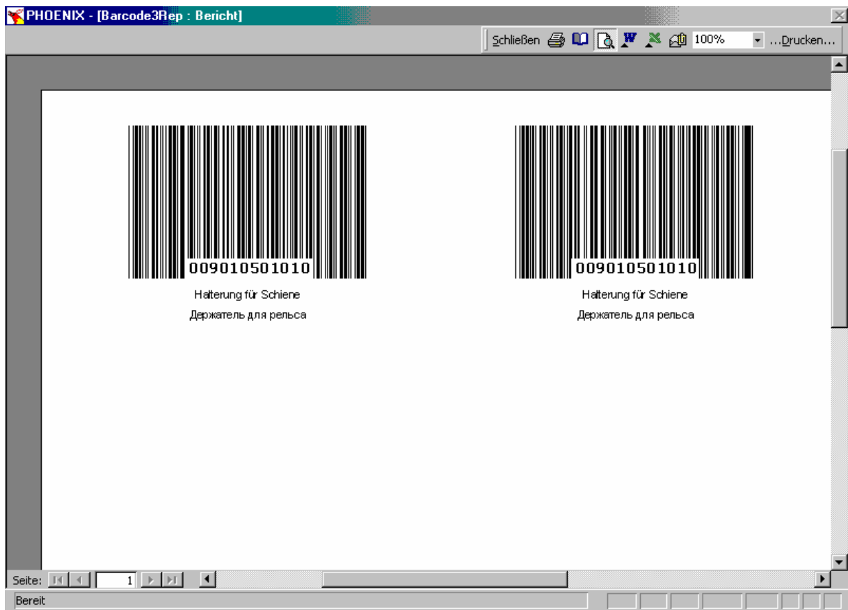
Abb. 22 Barcodedruck
