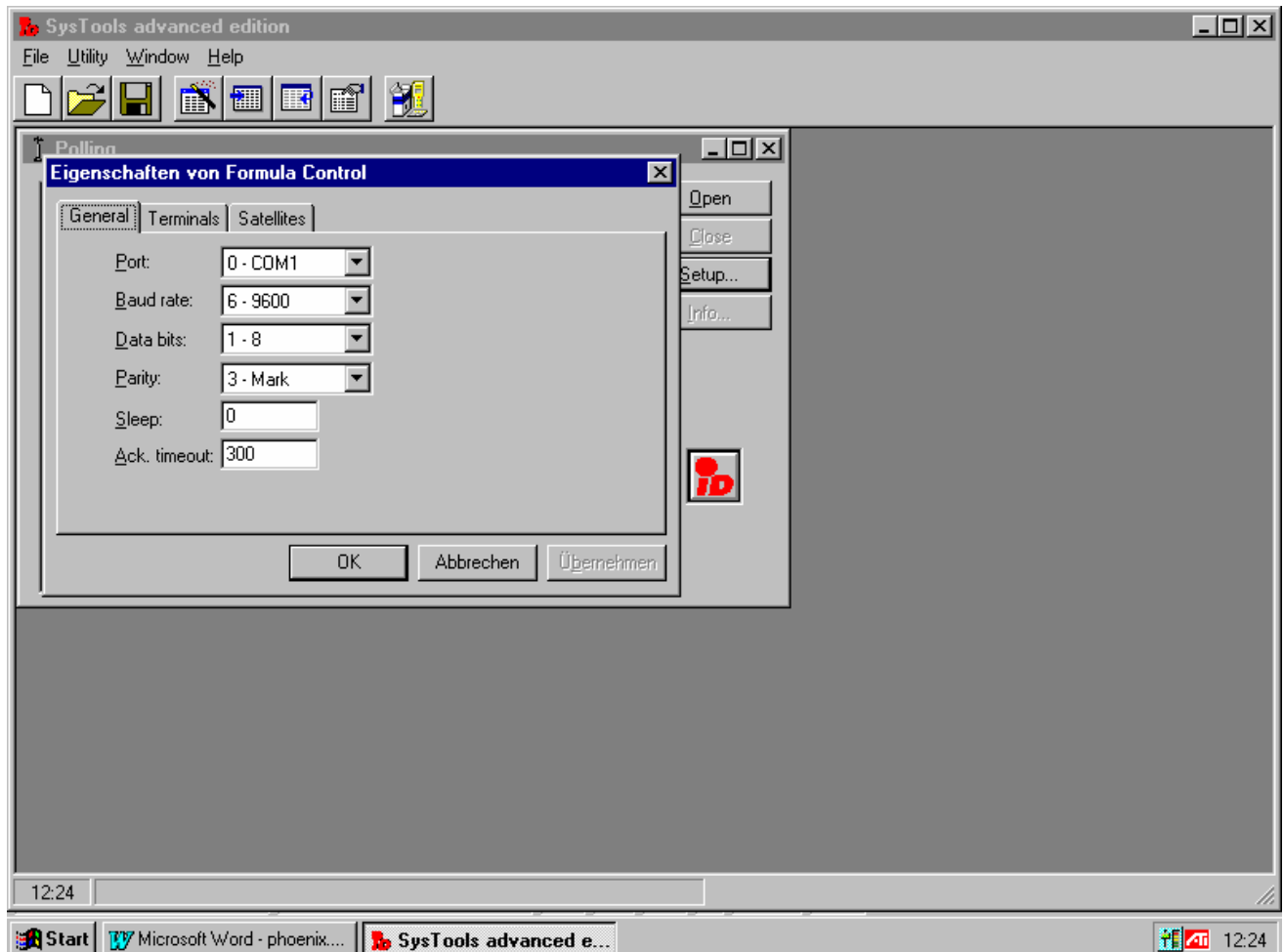
Abb. 44 Konfigurationsdaten
