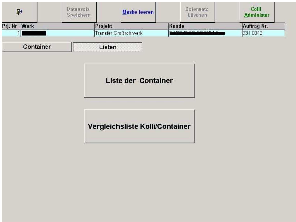
Abb. 33 Containerdaten
