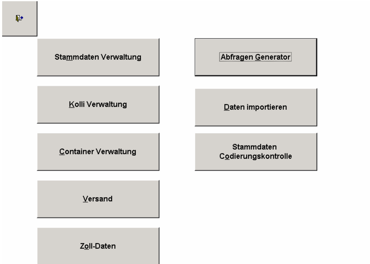
Abb. 25 Hauptmenü
